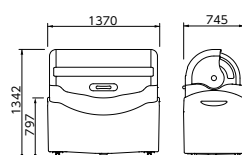
容量 約700ℓ
