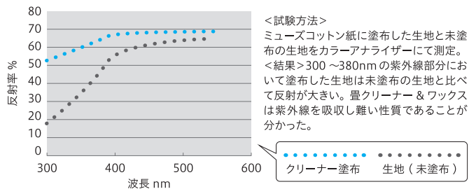
紫外線カット測定結果 紫外線 300～400nm
