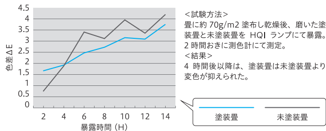
促進耐光性試験
